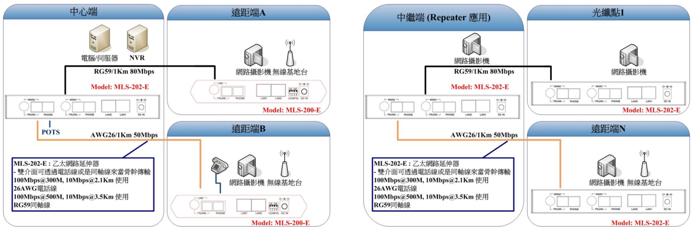
圖A: 點對點連接應用：遠距A、遠距B、中心端，三處網路利用電話線或是同軸線來達到網路互相連接目的。
